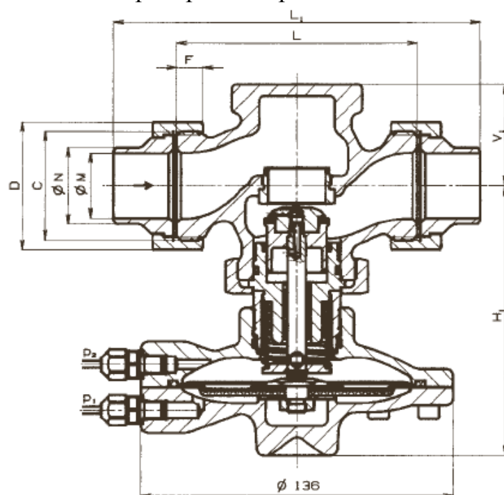
Вентили RD 122 D../W с приварным нарезным соединением.
