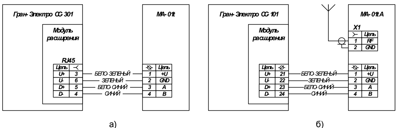
Рисунок 1. Схема подключения МА-01t к счетчикам электрической энергии «Гран-Электро СС-301» (а) и «Гран-Электро СС-101» (б).
