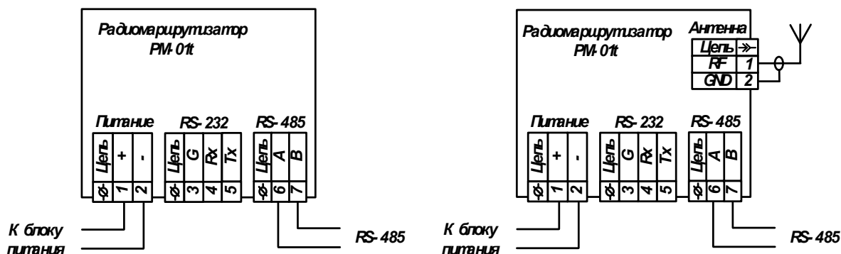
а) Радиомаршрутизатор РМ-01t со встроенной антенной
